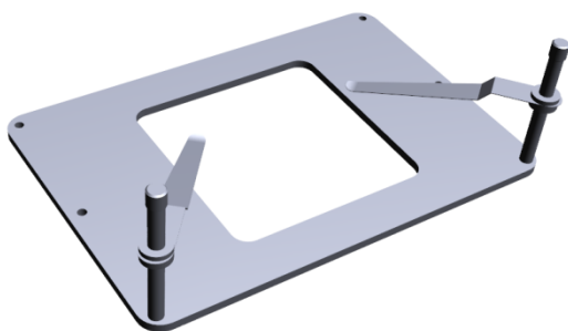
B00110 : DSH K ホルダ (FF □76 穴) B システム
